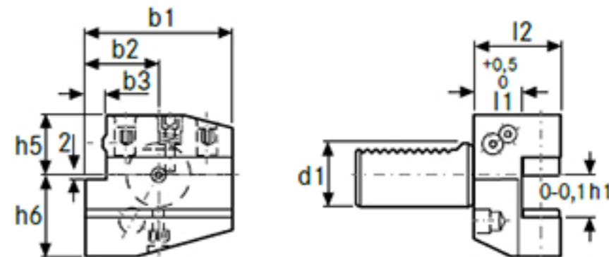
Porte-outil radial forme B2, côté gauche, court
