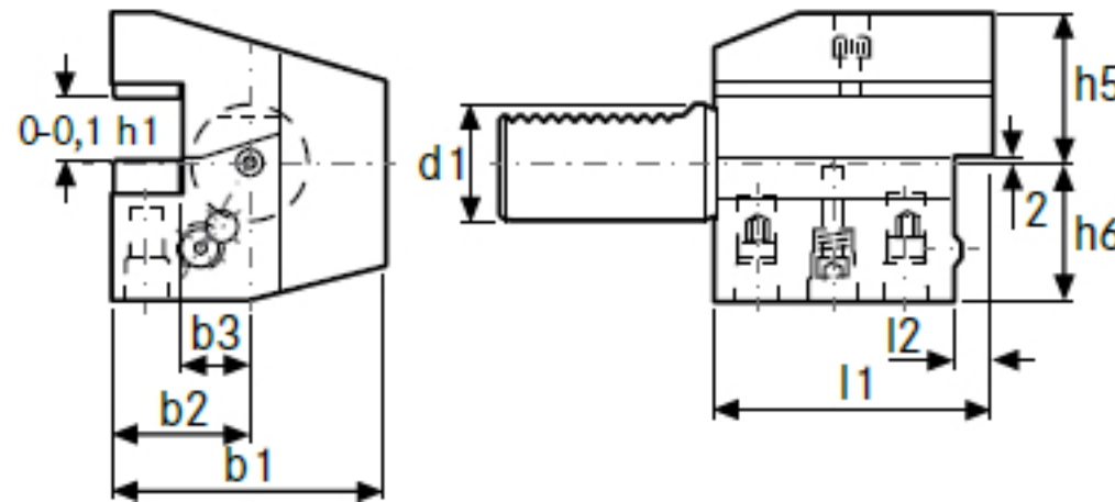
Porte-outil axial, forme C4, en hauteur, côté gauche
