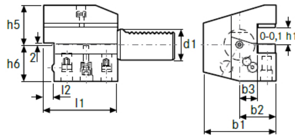
Porte-outil axial, forme C3, en hauteur, côté droit
