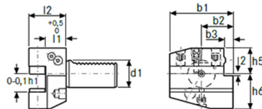
Porte-outil radial forme B1, côté droit, court
