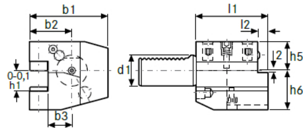
Porte-outil axial forme C2 côté gauche
