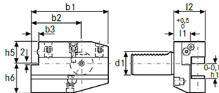
Porte-outil radial forme B6 côté gauche, long
