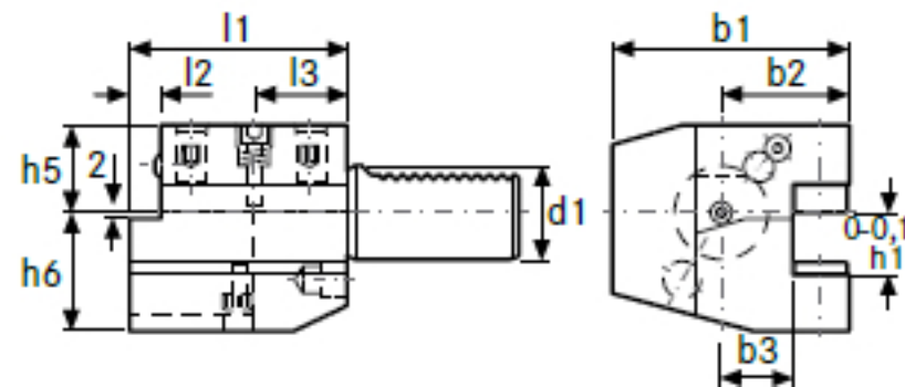
N° de réf. 001-003, 005-006 Porte-outil axial forme C1 côté droit
